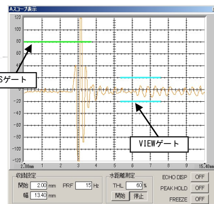
Aスコープ
