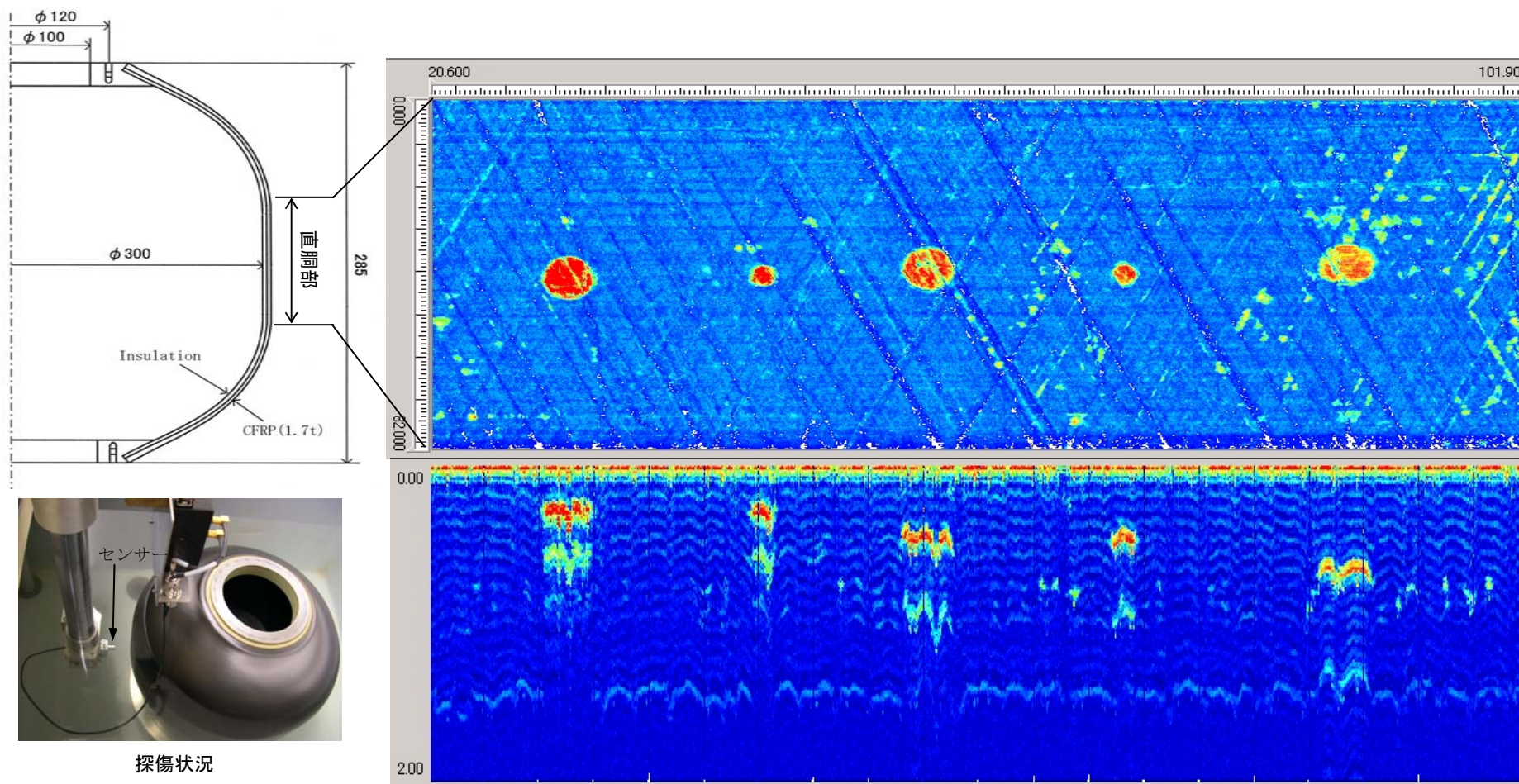
複合材圧力容器人工欠陥試験片の超音波探傷結果
